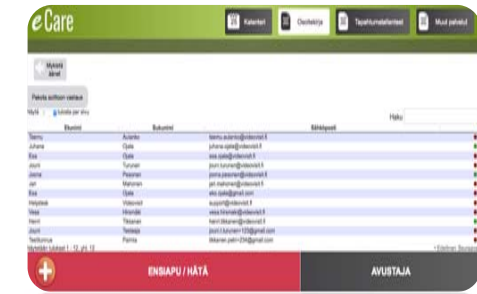
Ammattilaisen käyttöliittymä
